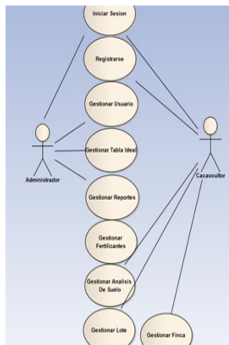
Figura 1. Casos de uso del Sistema y usuarios
