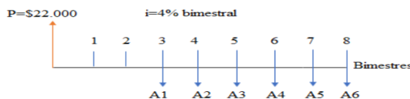
Figura 4: Diagrama de flujo ejercicio práctico 1
