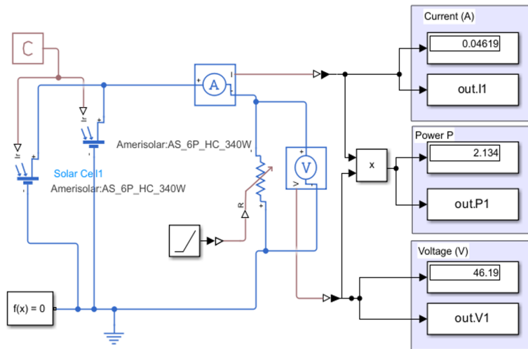
Fig 3: Diagrama de bloques simulink, arreglo de dos paneles solares Amerisolar de 340 \text{ W} .
