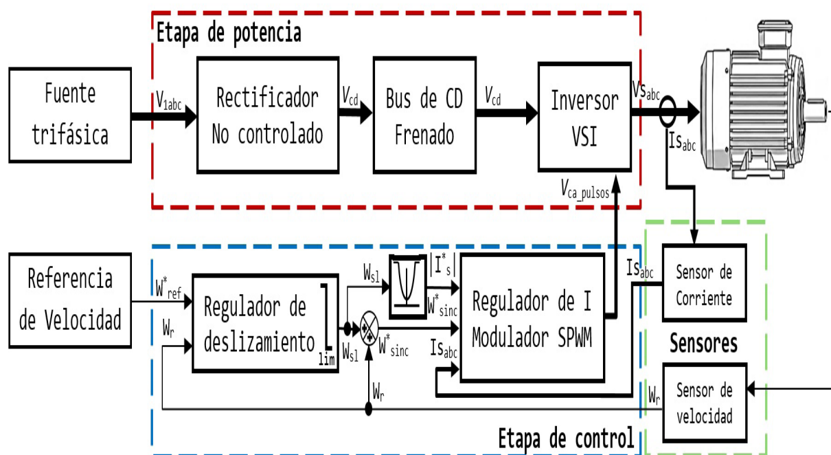
Figura 3 Diagrama de bloques del control escalar con inversor de voltaje del motor.
