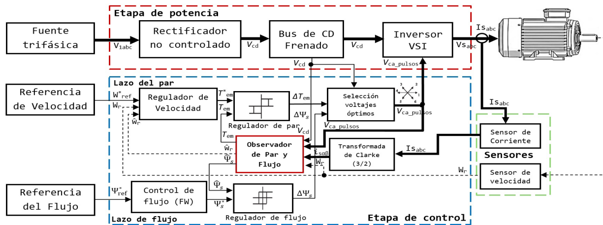
Figura 5 Diagrama de bloques del control directo del par del motor.
