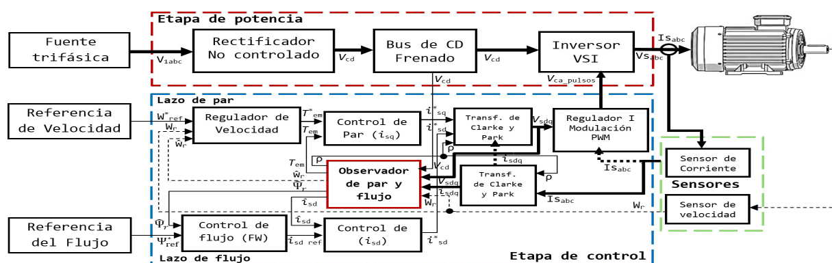
Figura 4 Diagrama de bloques del control vectorial por campo orientado directo.
