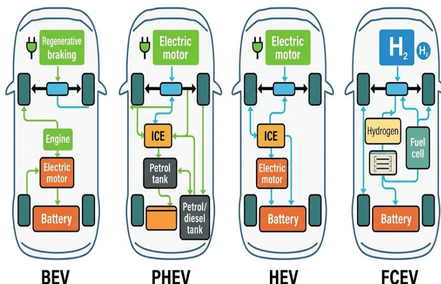
Figura 6 Comparativo de vehículos eléctricos Fuente: adaptación artículo [45].
