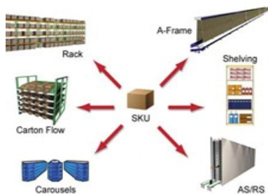
Ilustración 154. Slotting / Direcccionamiento
