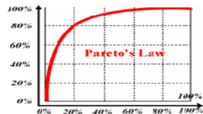
Ilustración 57. Pareto's Law / Ley De Pareto
