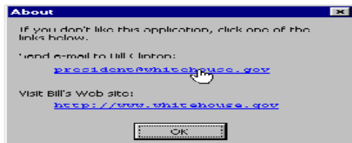
Ilustración 178. Hyperlink / Hipervínculo
