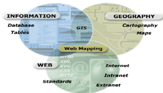
Ilustración 180. Mapping / Mapeo
