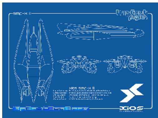
Ilustración 170. Blueprint / Huella
