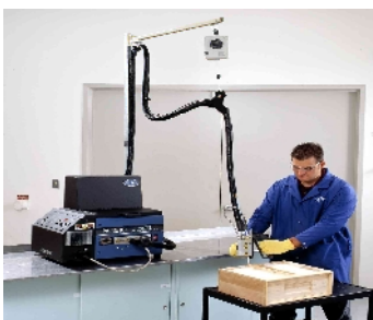
Ilustración 30. Assembly / Ensamble..
