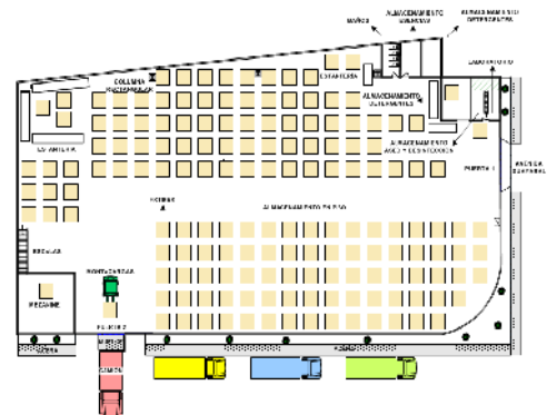
Ilustración 120. Layout drawing / boceto (dibujo) de la distribución física
